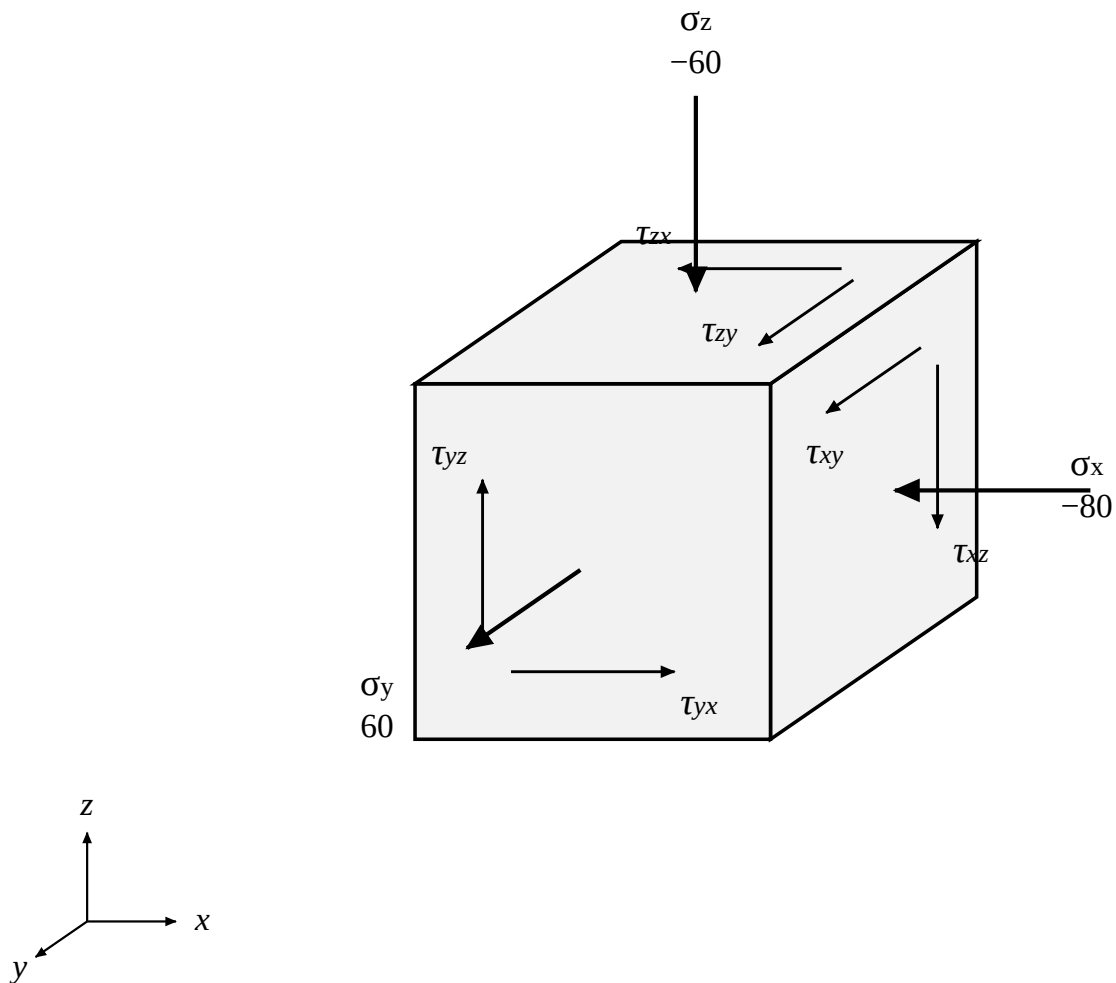
Рис. 1.1 — напряжения на гранях элементарного параллелепипеда, МПа. Оси: z вверх, x вправо, y на зрителя.
