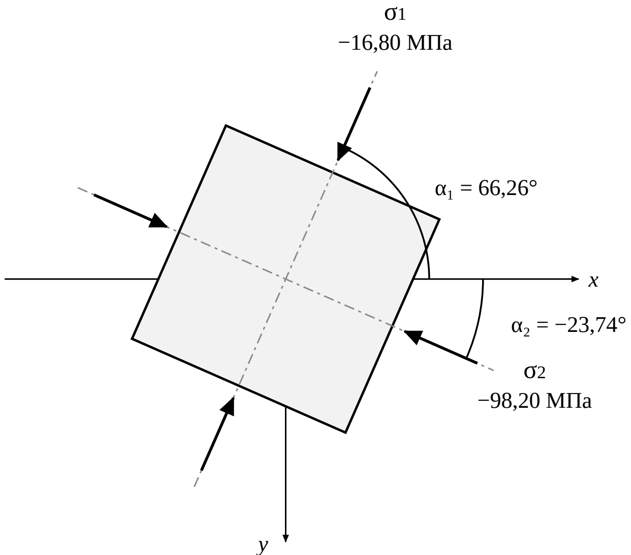
Рис. 2.3 — главный элемент: от оси x вверх отложен угол \alpha_1 = 66,26^\circ , перпендикулярно ему — направление \alpha_2 = -23,74^\circ . Оба главных напряжения сжимающие, поэтому стрелки направлены к граням.
